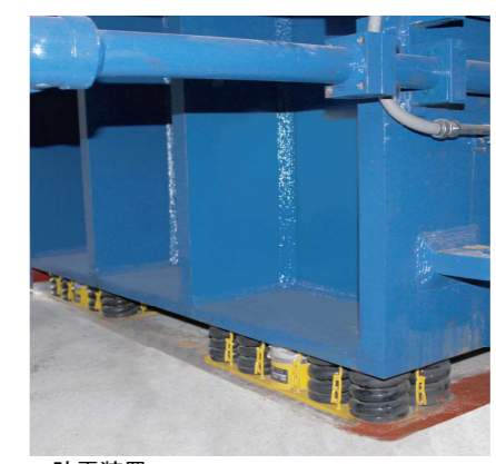
▲防震装置
