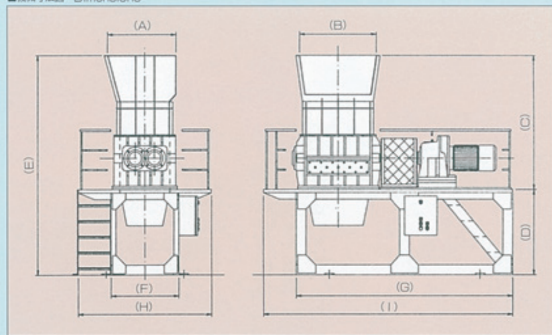
■機械寸法図 Dimensions
